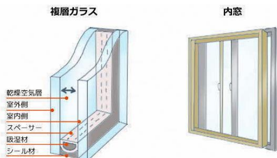
図 窓の断熱
