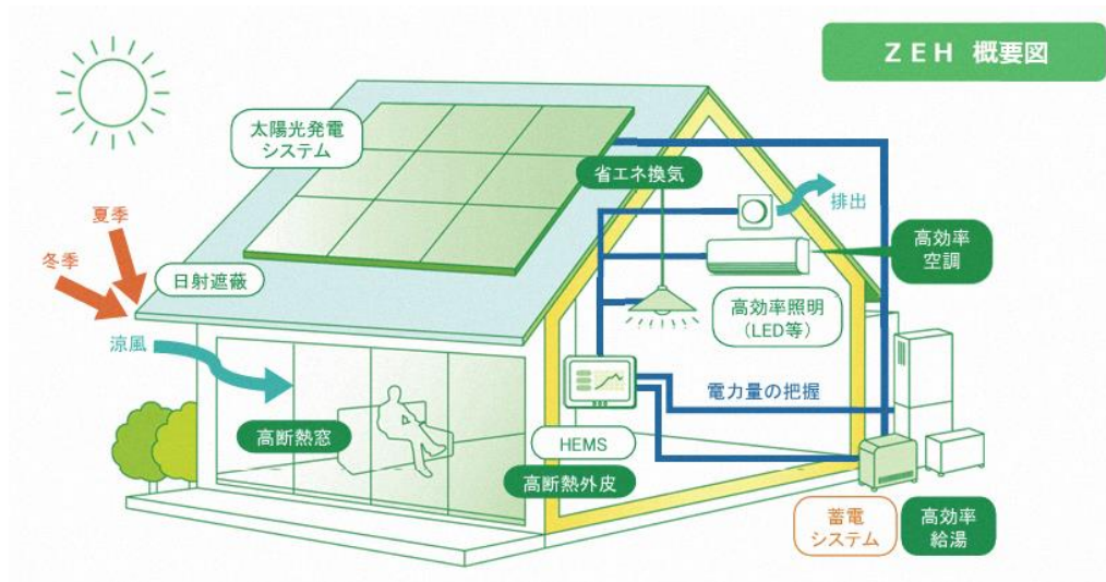
図 ZEH概要図
