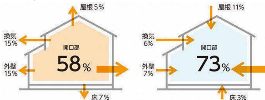
図 住宅への熱の出入り（左：冬の暖房時 右：夏の冷房時）
