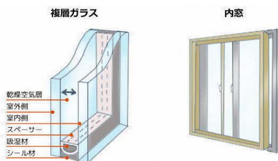
図 窓の断熱
