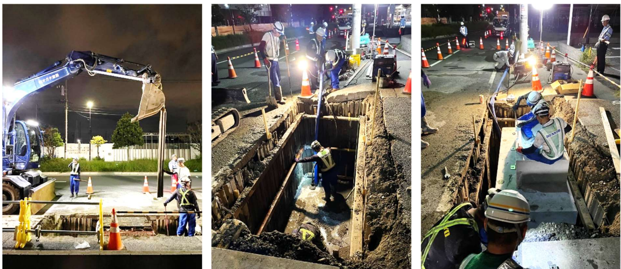
補助第251号線 実際の工事の様子
