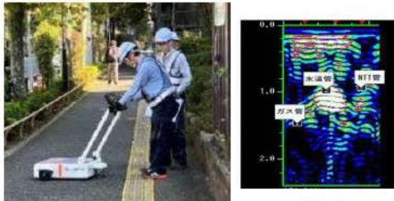
図：地中レーダー探査の様子
