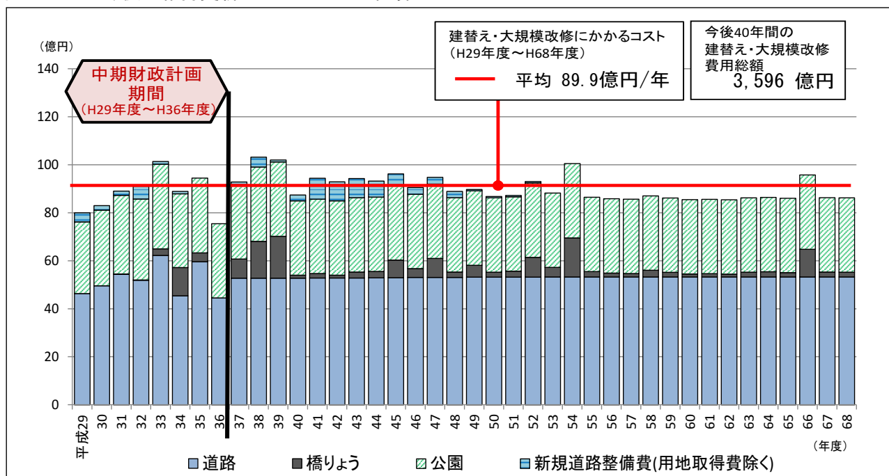
図5-4 今後の維持更新にかかるコスト試算
