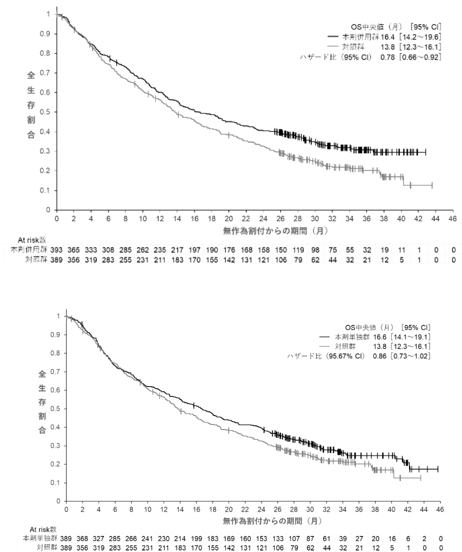
図1 OSのKaplan-Meier曲線
