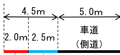
加平谷中トンネル (自転車歩行者道内での分離)
