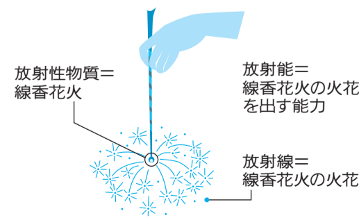
図1 放射性物質を線香花火に例えると
