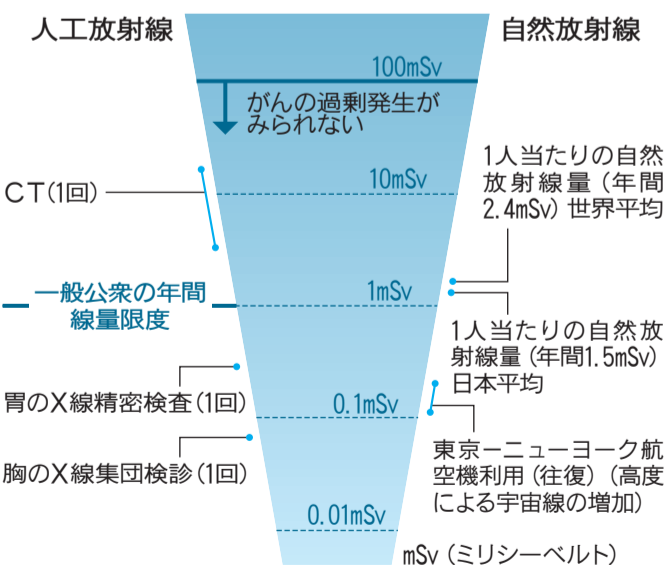
図2 日常生活で受ける放射線量
