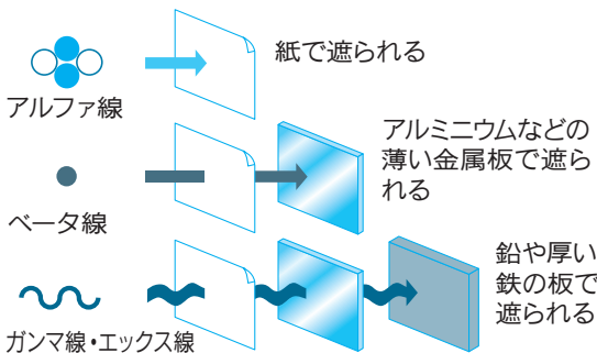
図1 放射線の種類とものを通り抜ける力
