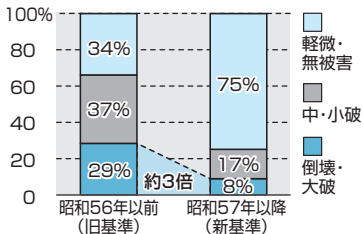
図1 阪神・淡路大震災の 建築年別の被害状況
