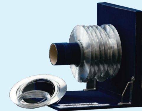
▲鏡のごとき切断面こそ切れ味の証(鏡面切り加工)。極細加工した金属が円盤になっている
