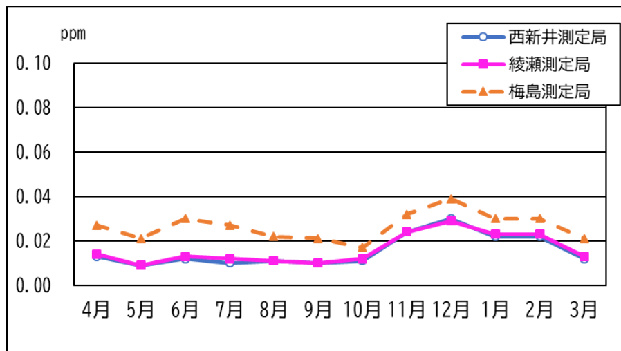
資 2-8 窒素酸化物（NO x ）月別变化
