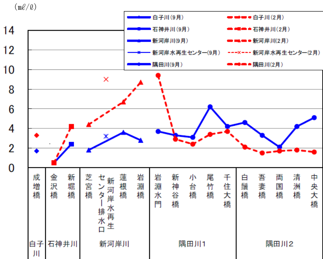
資 16-2 BOD縦断変化
