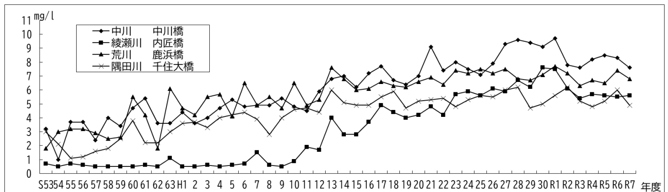
資13-3 DOの経年変化
