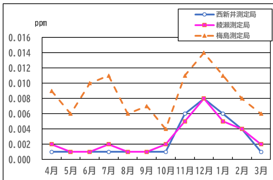
資 2-7 二酸化窒素（NO 2 ）月別变化
