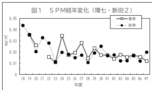
資 3-4 環状七号線の経年変化
