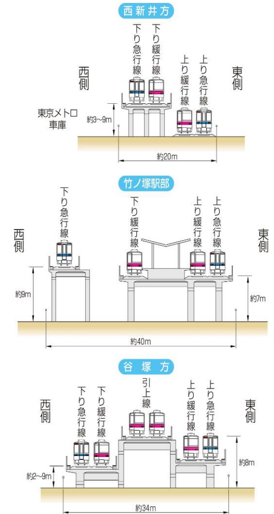
標準横断面図
