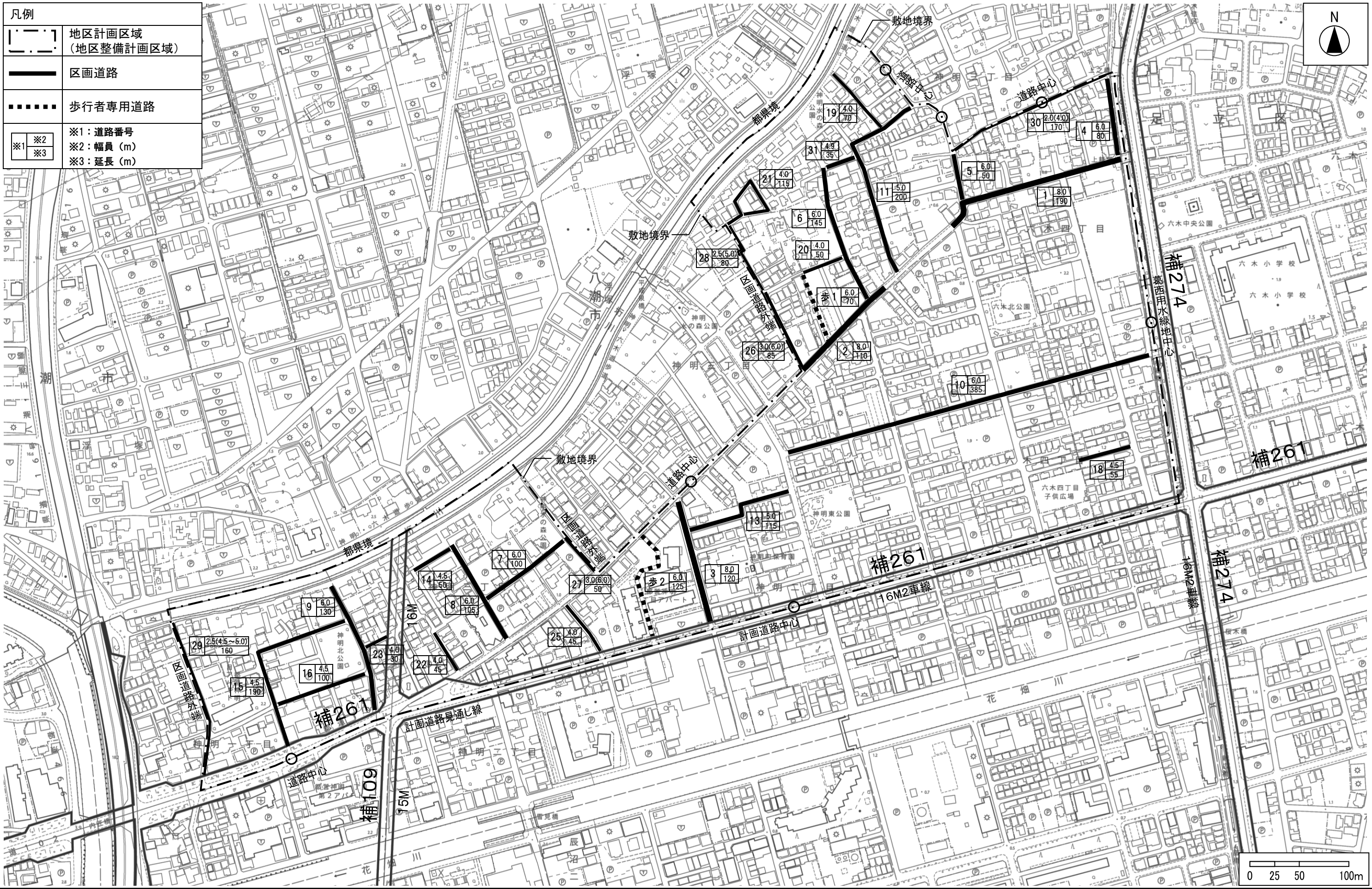
計画図 2
