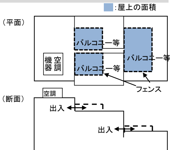
図C: 上部に庇等のないバルコニーなどを計画する場合
