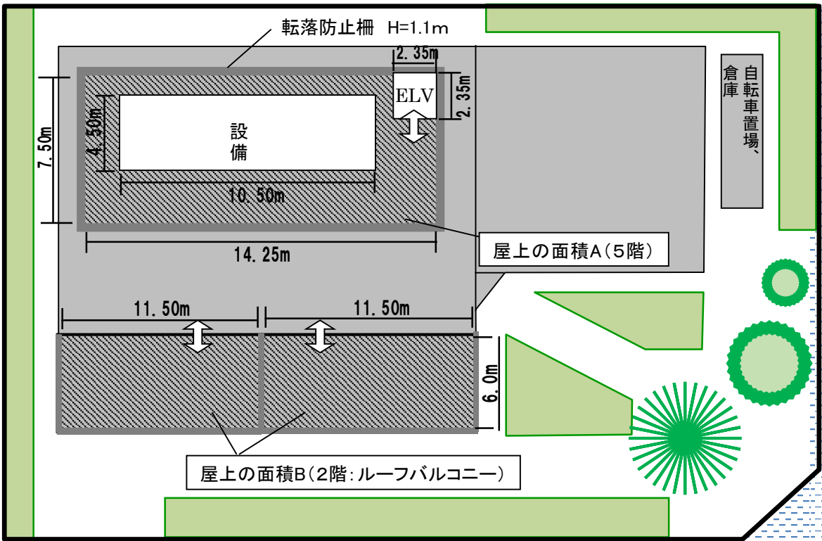
(才) 屋上平面図
