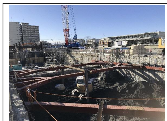
学校・寮棟：掘削工事
