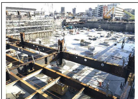
病院棟：地下躯体工事
