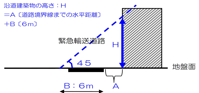
②前面道路幅員Lが12m以下の場合
