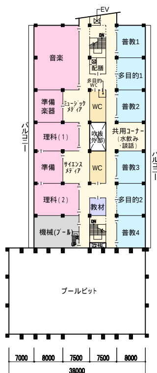
4 階平面図
