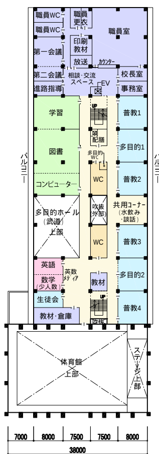
2 階平面図
