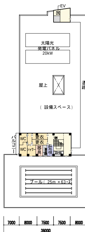
5 階平面図
