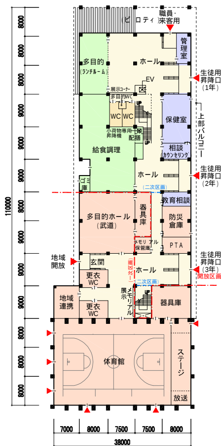
1 階平面図
