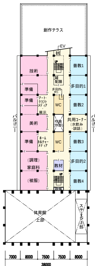
3 階平面図
