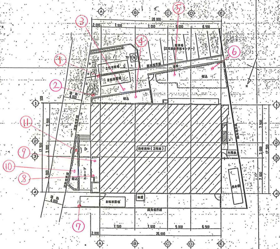
配座図 S. 1/200
