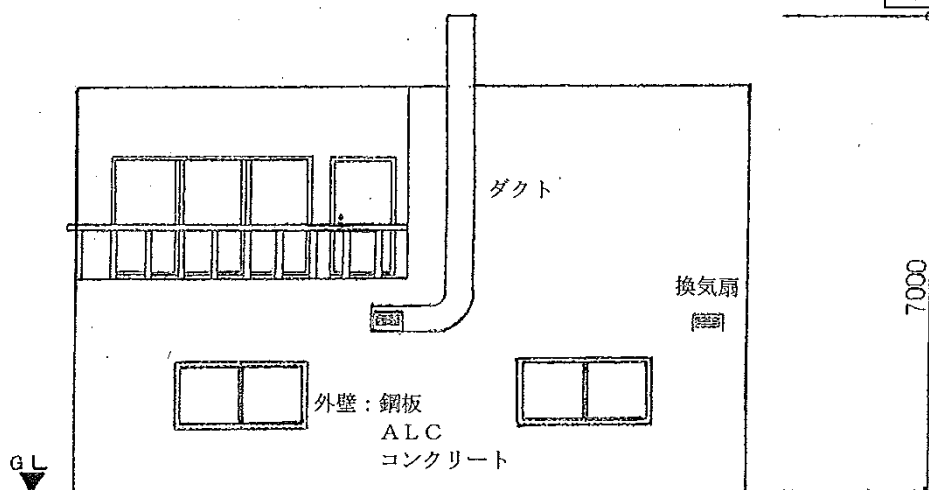
東立面図 1 : 100
