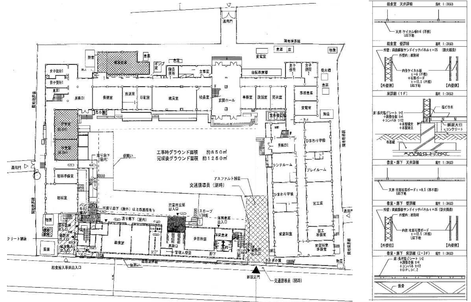
仮設校舎の天井、壁等の詳細図
