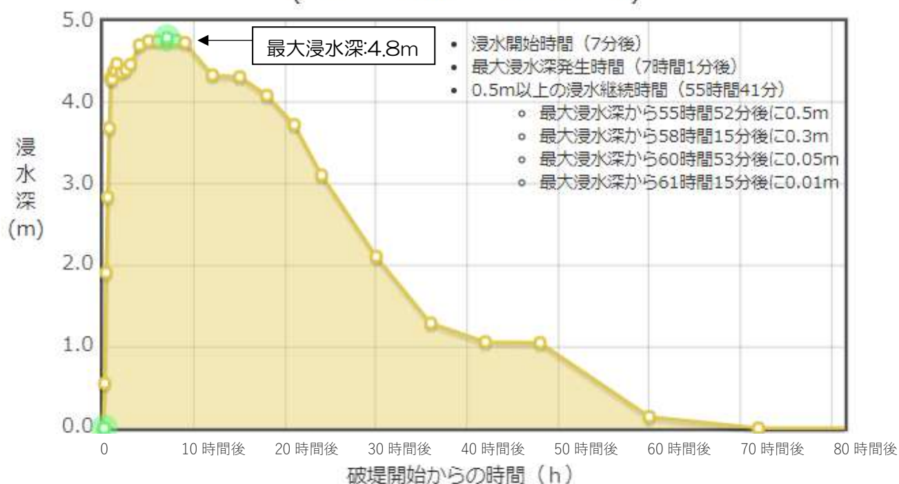
浸水シミュレーショングラフ（約 80 時間後まで） (BP284：荒川荒川右岸 16.50k)
