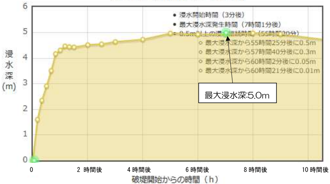
浸水シミュレーショングラフ (約10時間後まで) (BP286: 荒川荒川右岸 17.00k)
